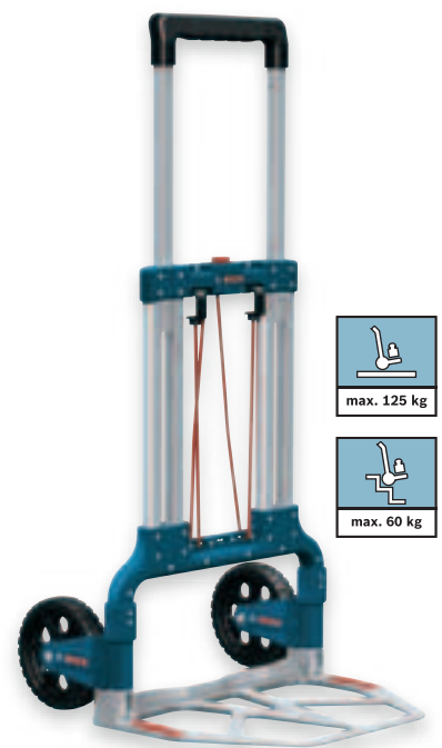
Diable en aluminium Référence : 2 608 438 021
